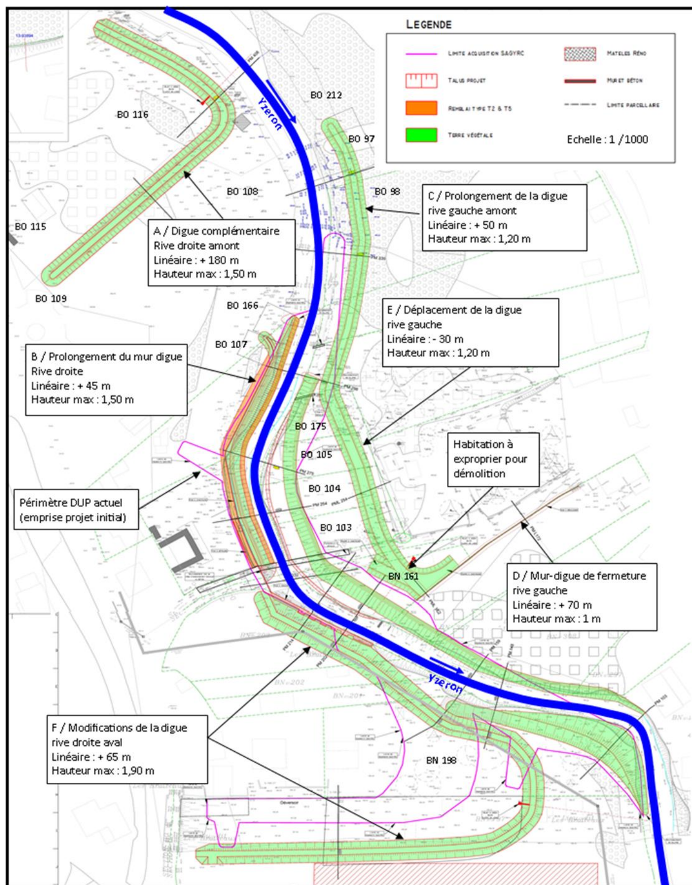
Figure 3 : localisation des aménagements modifiés au droit du gué de Ruelle Mulet à Francheville
