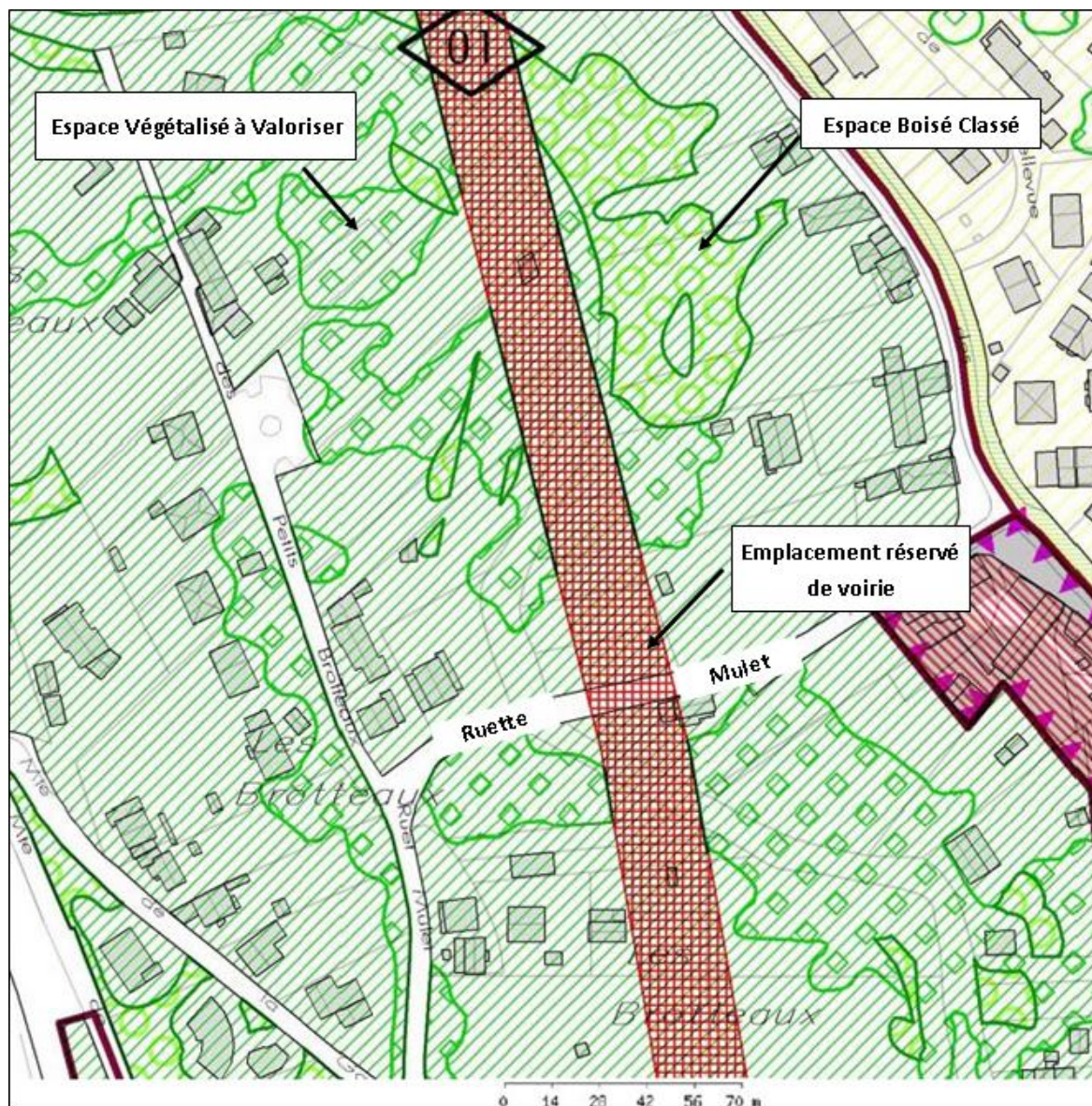
Figure 4 : Extrait du plan de zonage 1/5000 du PLU-H sur la commune de Francheville secteur de Ruette Mulet.
